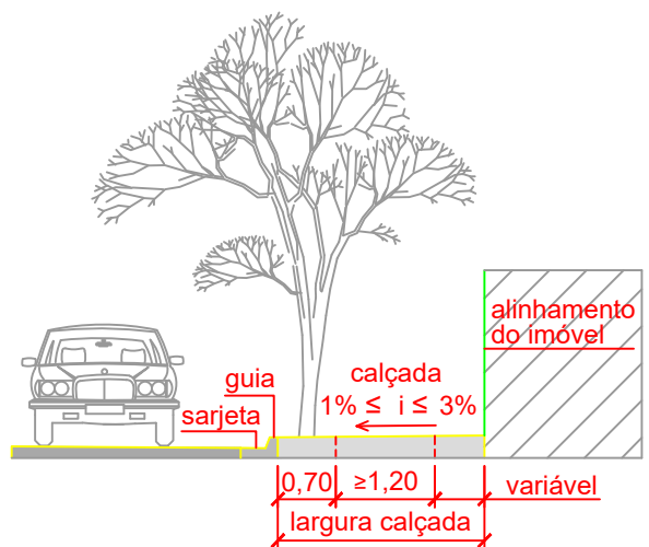
CORTE TRANSVERSAL
